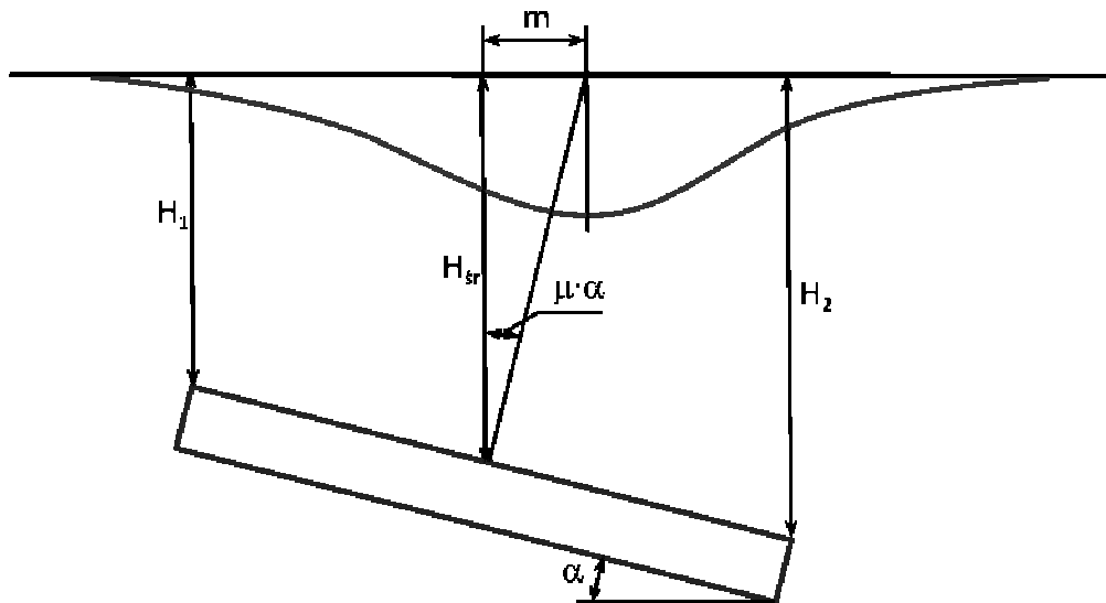
Rys.1. Efekt dewiacji wpływów w kierunku upadu warstwy złożowej [4]
