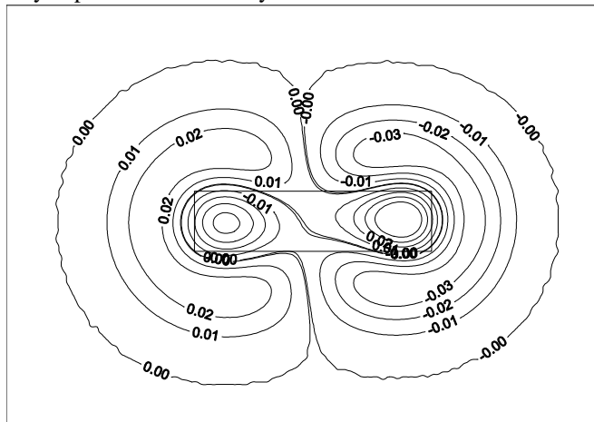
Rys. 5. Różnica pomiędzy obliczonymi obniżeniami Fig. 5. Difference between calculated subsidence
