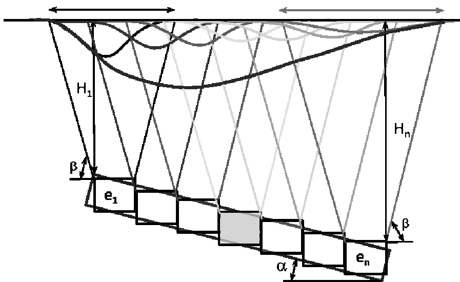
Rys.2. Efekt asymetrii niecki obniżeniowej [4] Fig.2. Asymmetry effect in subsidence trough [4]
