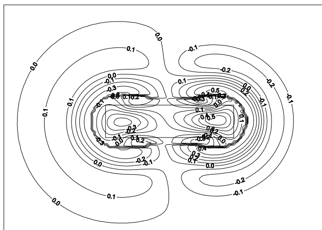
Rys. 6. Różnica obliczonych maksymalnych odkształceń poziomych Fig. 6. Difference between calculated maximal horizontal strains
