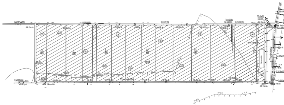
Rys. 4. Ściana eksploatacyjna uwzględniona w obliczeniach Fig.4. Exploitation panel considered in the subsidence prediction.
